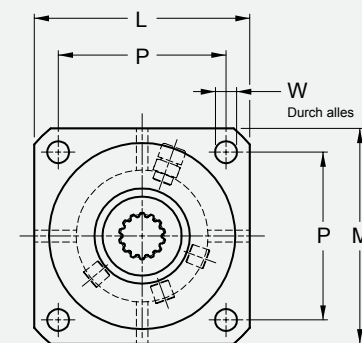
SAE C - 4 SCHRAUBENLOCH
