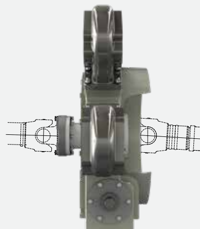
MPD mit KARDANWELLE IM EIN- ODER AUSGANG (MIT FUßMONTAGE)
